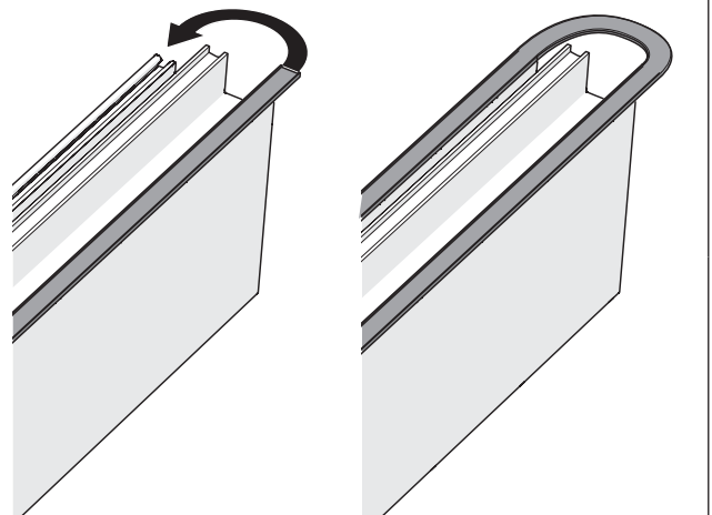
19 Schneiden Sie die Gummileisten auf zweimal die Länge des Trägers +10 cm zu. Schieben Sie die Gummileisten an der Wandseite mit einer Schlaufe in den Träger.
